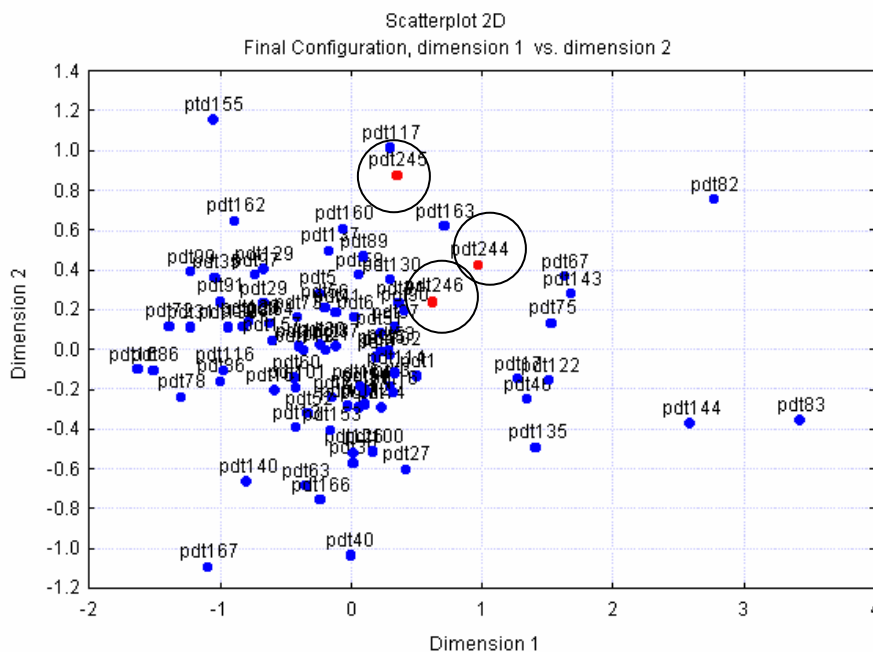
Figura 1: Configurazione in due dimensioni delle grappe esaminate
