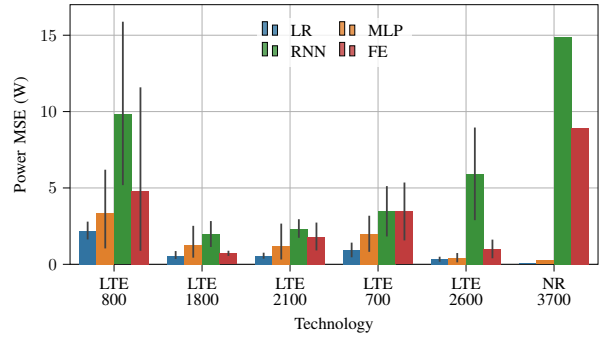
(b) MSE
